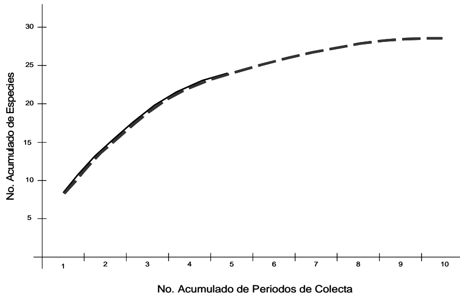
Figura 2. Curva de acumulación aleatorizada observada (—SACumAleat) y curva de acumulación esperada (----- SACumEsp) de acuerdo al modelo de Dependencia Lineal.
